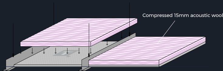
Scénario 2: Installation with compressed acoustic wool above the T|Karra tile.
